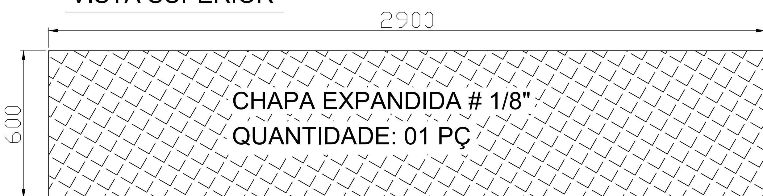
VISTA SUPERIOR
