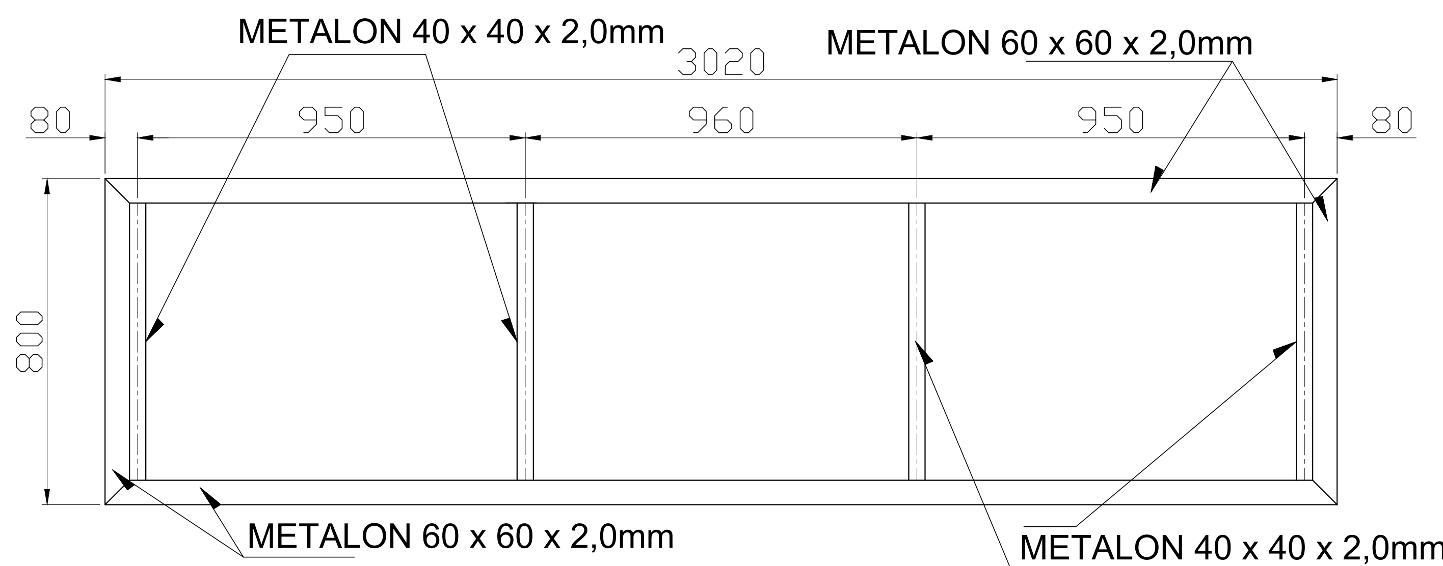
VISTA SUPERIOR
