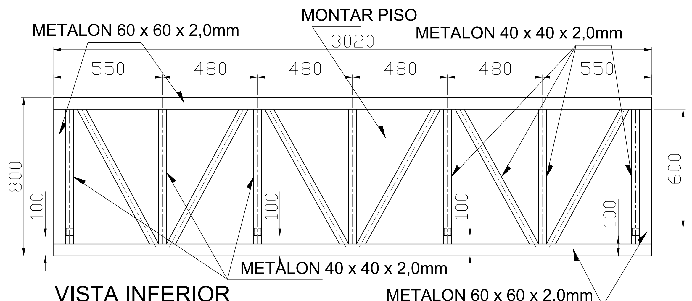
VISTA INFERIOR
